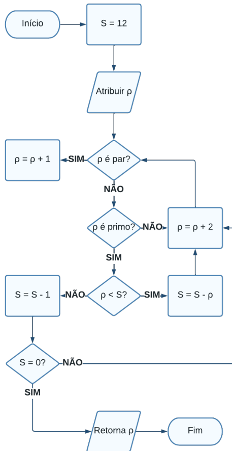
Fluxograma 1 – Exemplo de fluxograma de algoritmo
